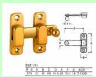
扉開放防止・掛け金 家具扉の開放防止金具として、もっともベーシックな、掛け金です。扉の前につけて、使用します。
